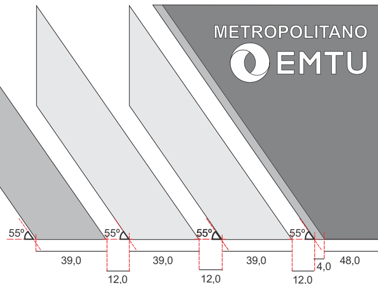
Faixa Metropolitano - Diagramação Micro-ônibus e Mini-ônibus
